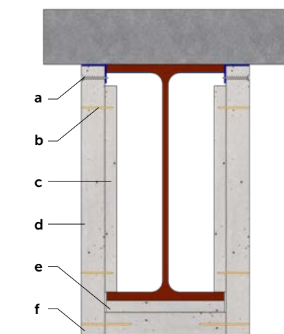
MED 1 PLATELAG Bjelkehøyde inntil 600 mm.
